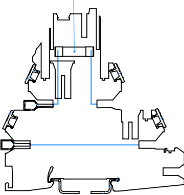
SECTION B-B SCALE 1 : 2
